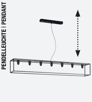
70717 ↔ 130x18 cm / ↓ 150 cm excl. 7 x E14 - max. 10 W
