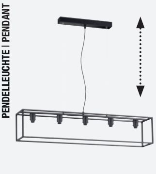
70594 ↔ 95x18 cm / ↓ 150 cm excl. 5 x E14 - max. 10 W
